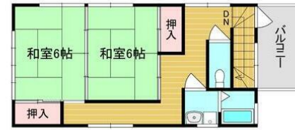
2階平面図
